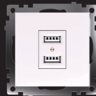
Розетка USB 2-местная Размеры А*В*Н, мм (55x35x53)
