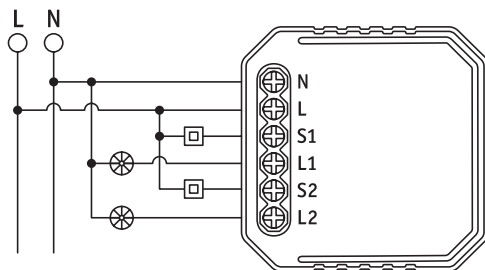
Схема подключения
