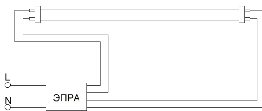
Светильник с ЭПРА до замены
